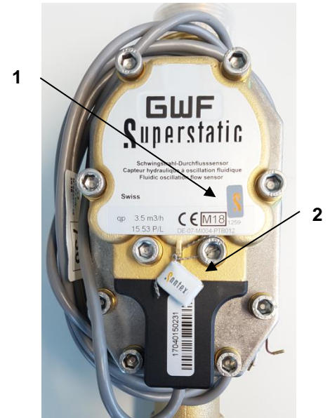
Eichplobmen / Calibration seals Ab Werk plombiert - Ex factory sealed 1: Klebplombe / Sticker seals 2: Drahtplombe / Wire seal
